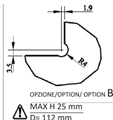
Dimensione Taglio Piano (Mm) Cut - Out Dimensions (Mm) Ausschnittmaße (mm)
